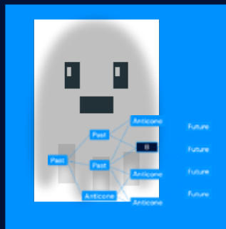
GhostDAG Protocol
