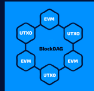
UTXO-EVM Interoperability
